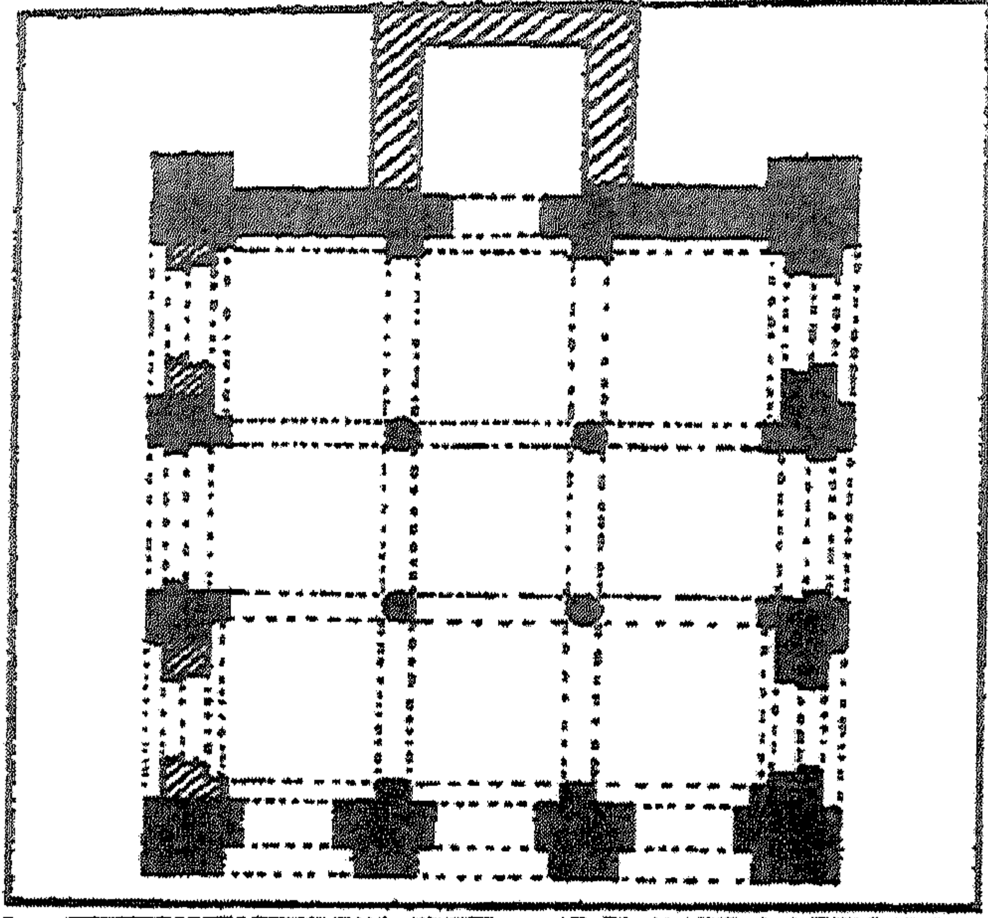
(شكل رقم ٣٥) رسم تخطيطي لمسجد البياض المرموم عن جولفان .
